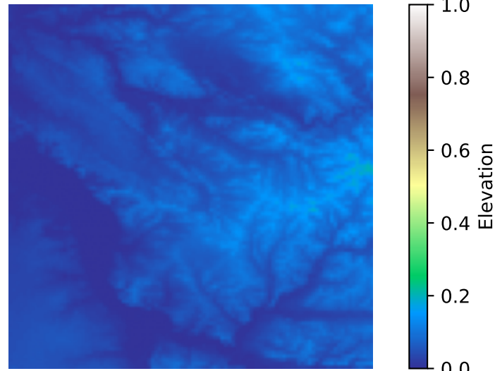
DEM
